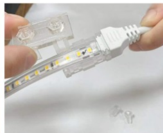
STEP 4 把接头上盖安装在接头下盖上
