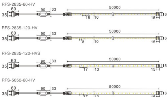
产品外形俯视图
